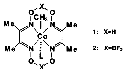
Fig. 1. Methyl(L)cobaloxime ( 1 ) and Methyl(L)BF 2 -cobaloxime ( 2 ).
